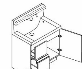
引出タイプ VJHK-755SYN-G/LM2H
